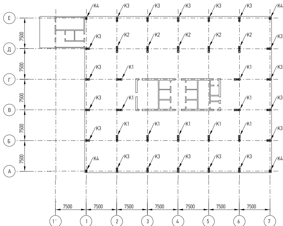
Рисунок 5.10 Монолитный железобетонный каркас с безбалочной системой перекрытия при сетке 7,5х7,5 м. Маркировочный план пилонов на уровнях 3-19
