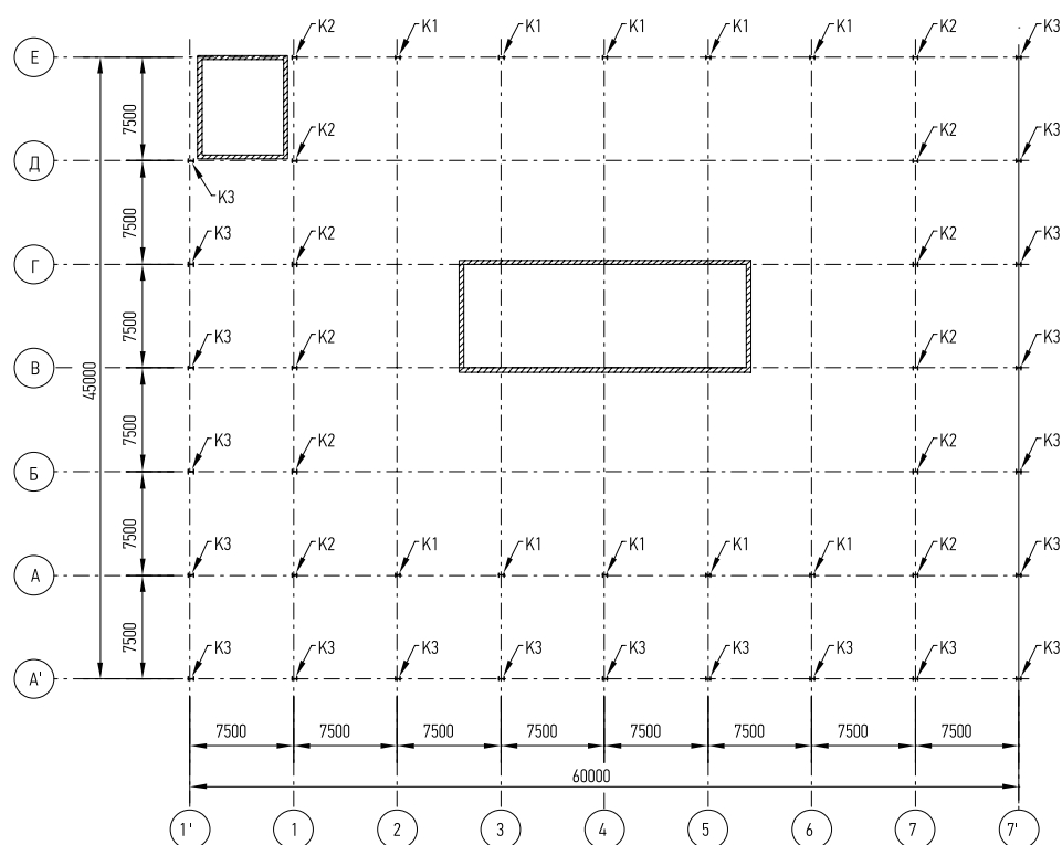
Рисунок 5.12 Вариант каркаса с применением стальных конструкций при сетке 7,5х15 м. Маркировочный план колонн
