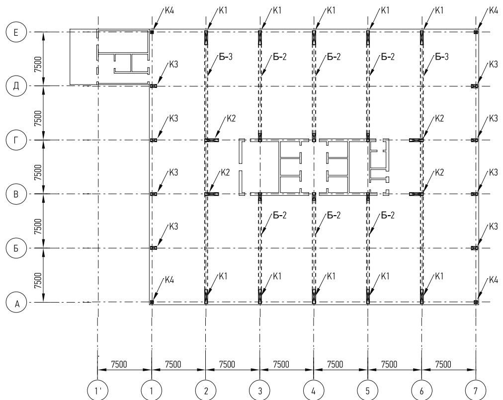
Рисунок 5.20 Монолитный железобетонный каркас с балочной системой перекрытия при сетке 7,5 х15 м. Маркировочный план несущих конструкций на уровнях 3-19
